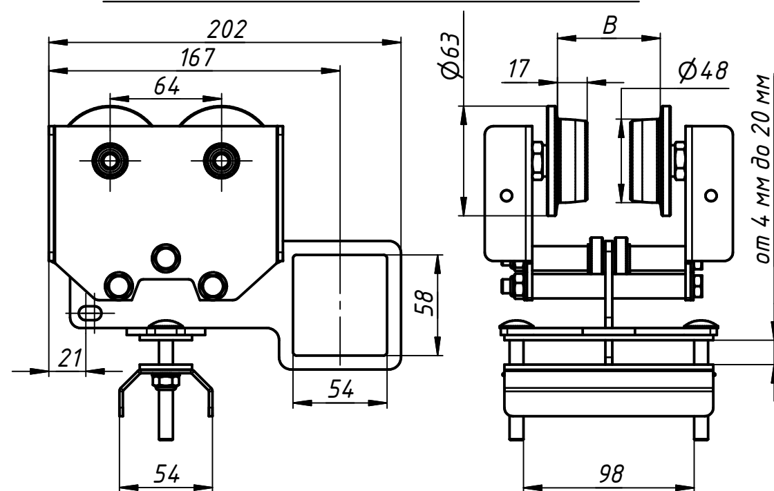
Кабельная тележка поводковая КТП-35(4)-02
