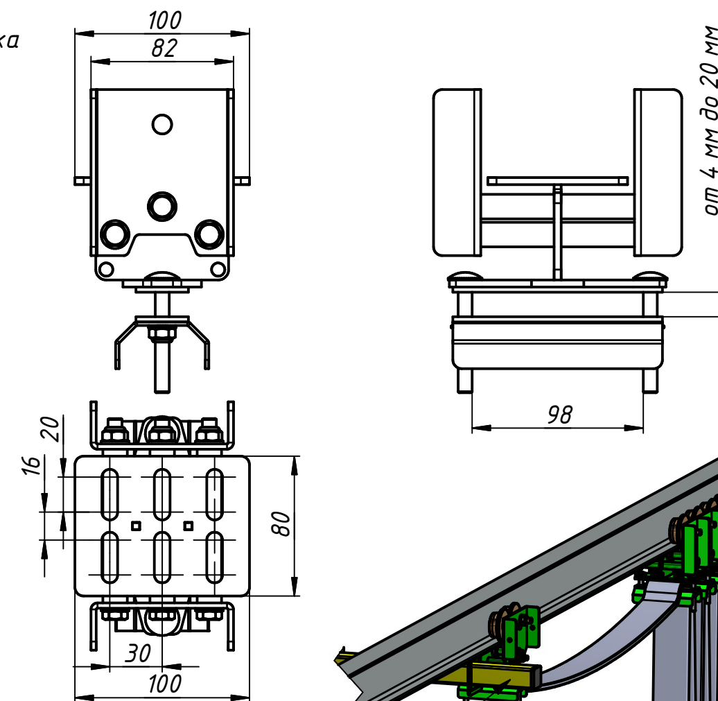
Кабельная тележка стационарная КТС-35-03
