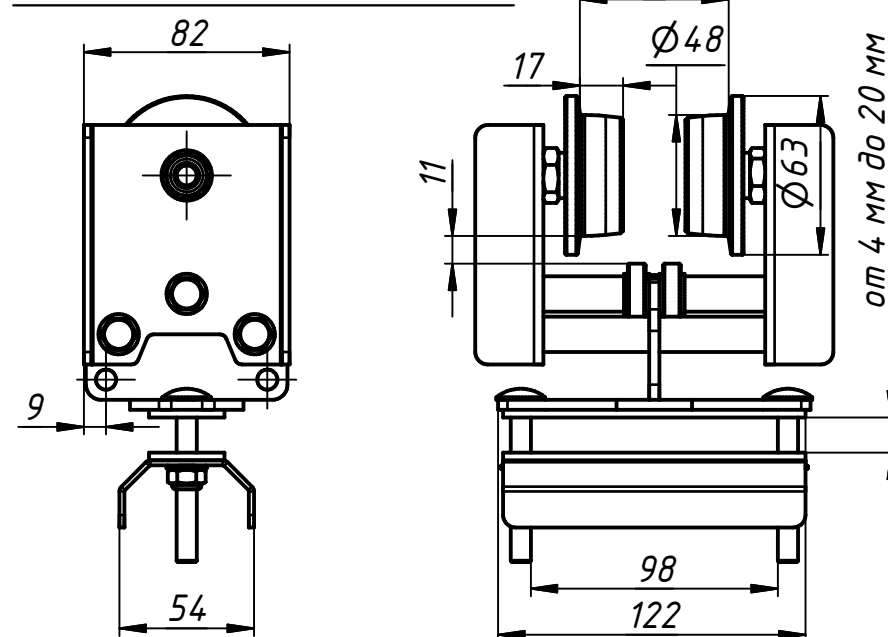
Кабельная тележка КТ-35-01
