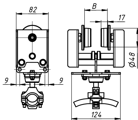
Кабельная тележка КТ-36-001
