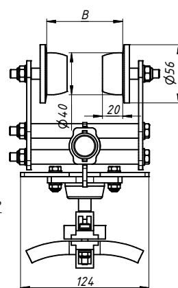
Кабельная тележка КТ-40-001
