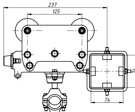
Кабельная тележка поводковая КТП-40-02
