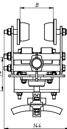
Кабельная тележка поводковая КТП-40-02
