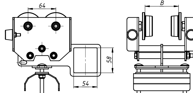
Кабельная тележка поводковая КТП-45-002
