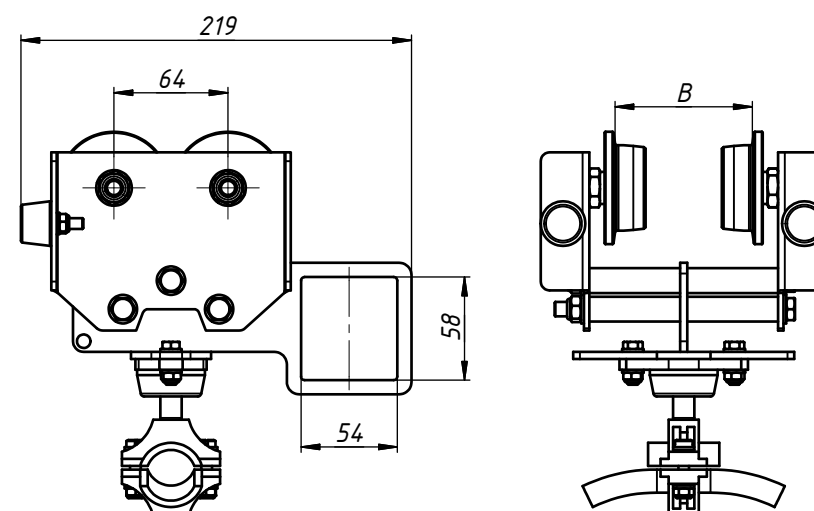
Кабельная тележка поводковая КТП-46-02
