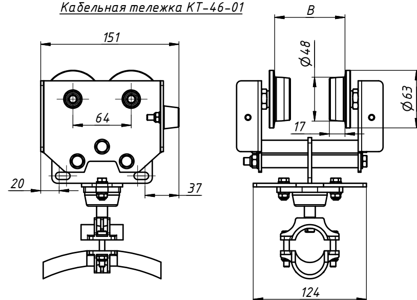
Кабельная тележка КТ-46-01
