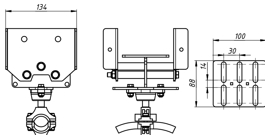
Кабельная тележка стационарная КТС-46-03
